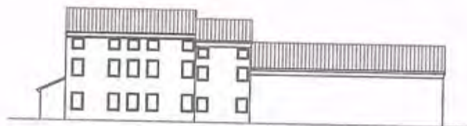
PROSPETTO NORD
